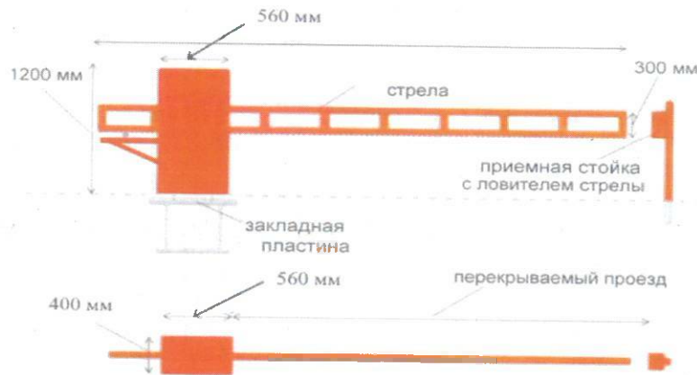
Рис. 2. Габаритные размеры
