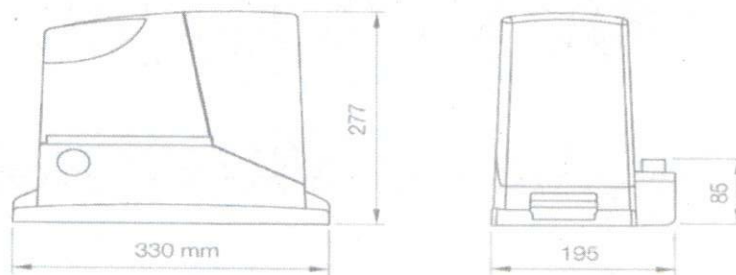
Внешний вид и габаритные размеры привода
